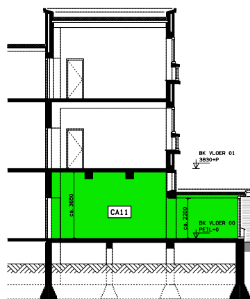
DOORSNEDE
