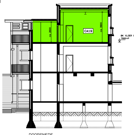
DOORSNEDE
